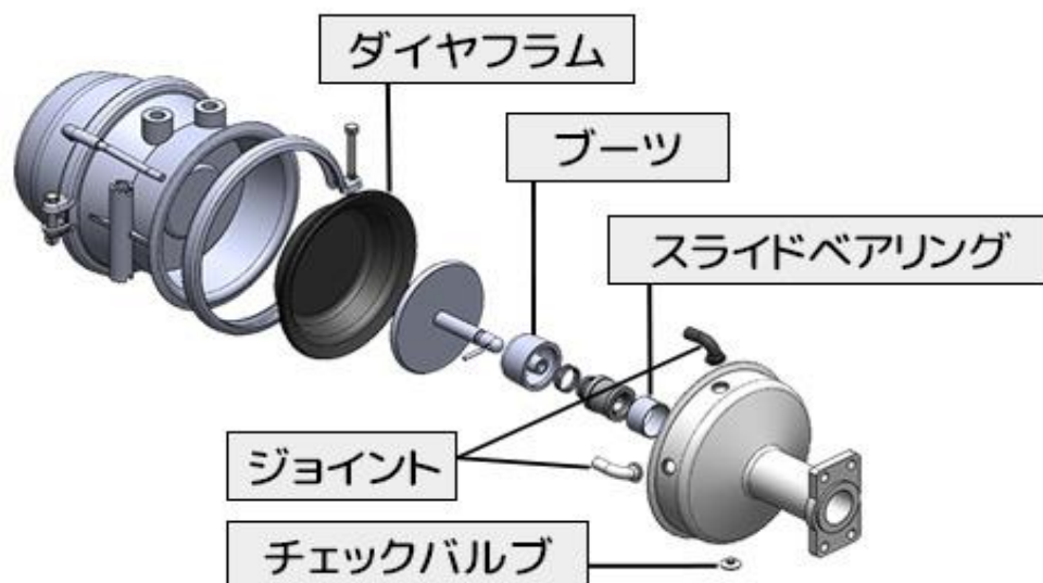
チャンバーキット取り付け図
