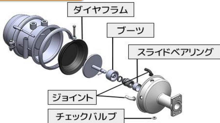
チャンバーキット取り付け図
