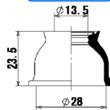
形状図
