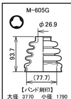
形状図
