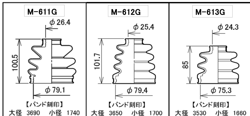
形状図
