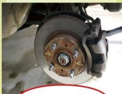
ブレーキローター
