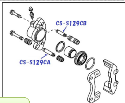
スライドピンシリンダー 取り付け図
