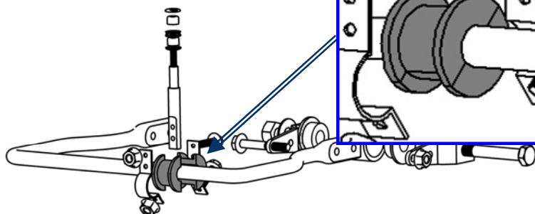
拡大図
